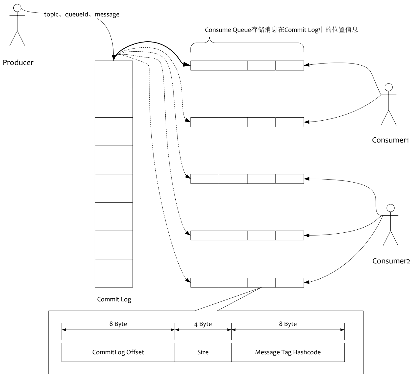
图表 7-1 RocketMQ 队列
